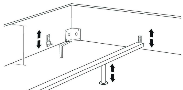
Einlegetiefen
